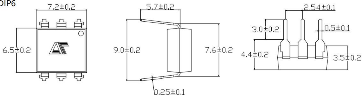
DIP6-M
