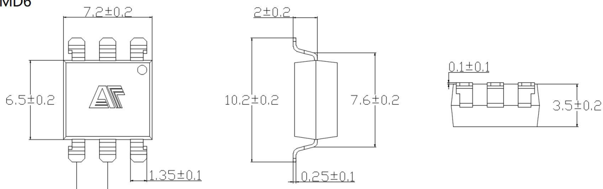
SMD6
