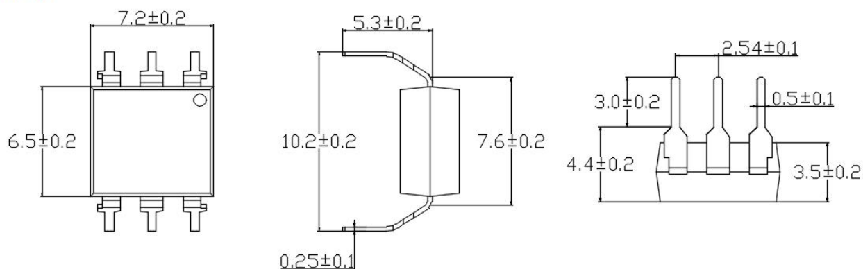
SMD6
