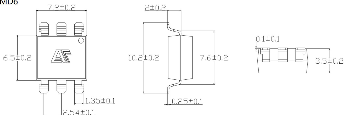
SMD6
