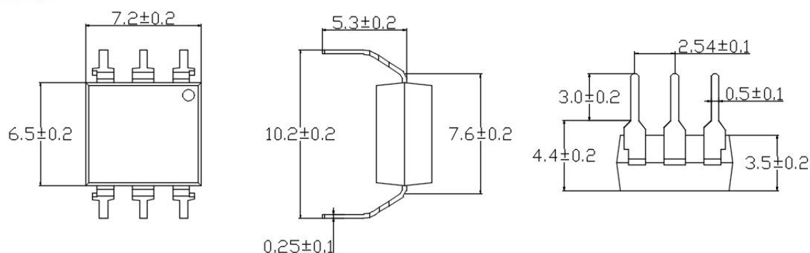
DIP6-M
