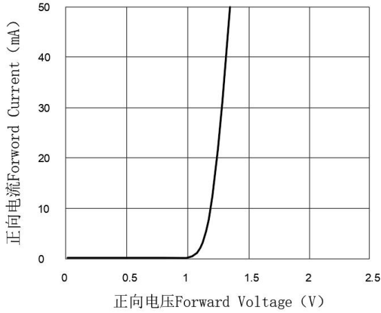
正向电压与正向电流特性曲线 Forward Current vs Forward Voltage
