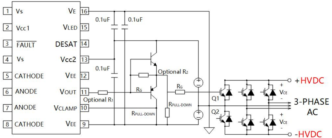
图.40 具有负栅极驱动，外部增压器的大型 IGBT 驱动。用于更高功率应用的 VCLAMP 控制二级放电路径
